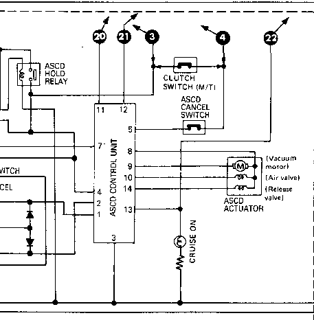
(VG30E engine model)
